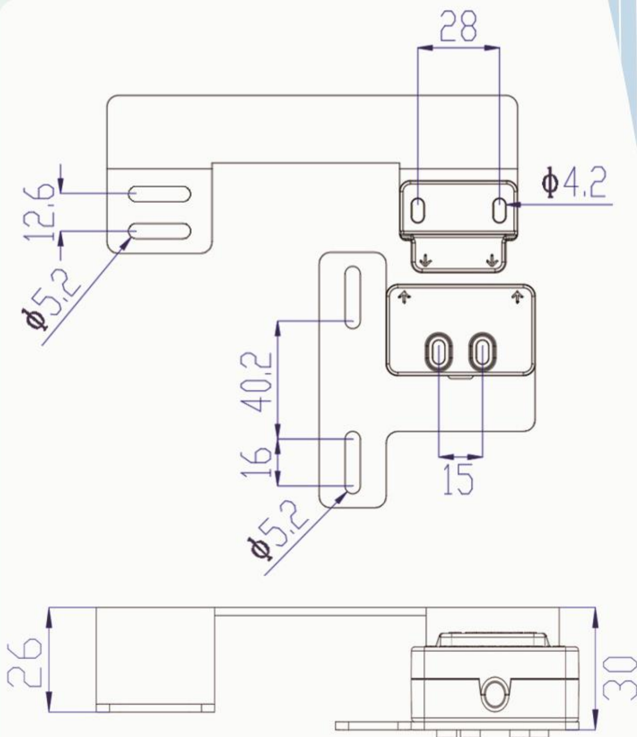
主门锁示意图 Main lock
